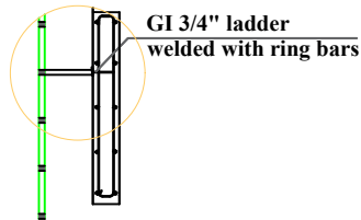
Detail(B-B)
